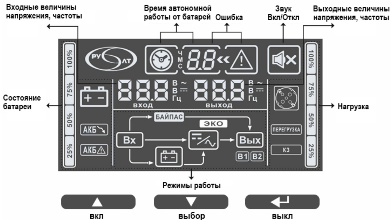
Рисунок 2. Передняя панель ИБП.
